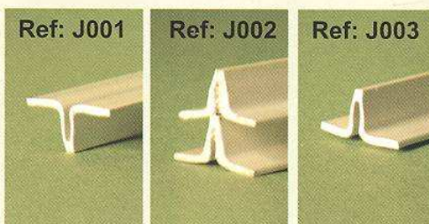
Tipos de junquillos para realizar las juntas entre paños de pavimento.
